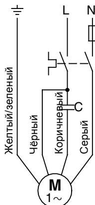
Рис. 13 Электродвигатели фирмы Franklin
