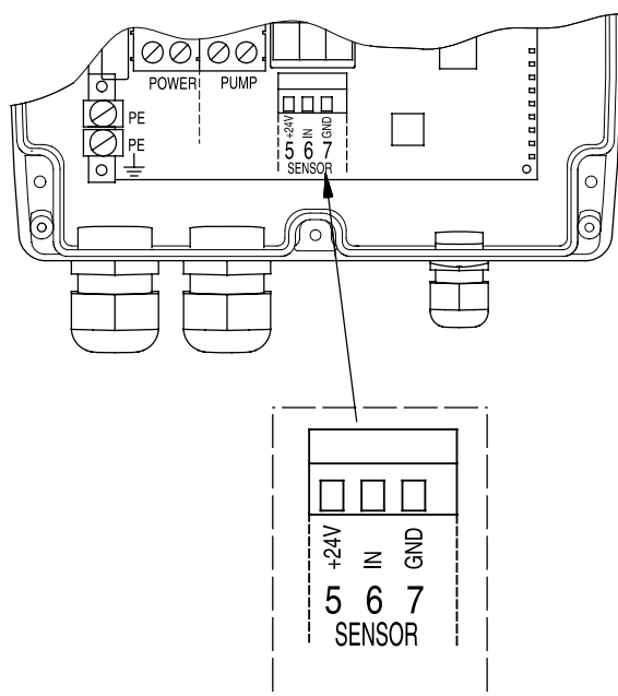
Рис. 37. CU 301 подключение.
