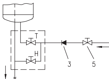
Open (niet onder druk staand) systeem
