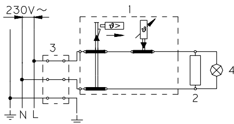
Az elektromos kapcsolás vázlata
