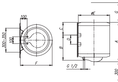
Anslutnings- och monteringsmått av varmvattenberedaren [mm]
