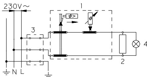
Schéma elektrické připojky
