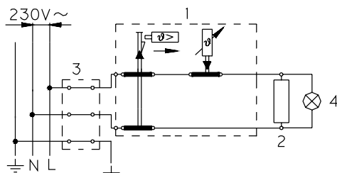
Электросхема
