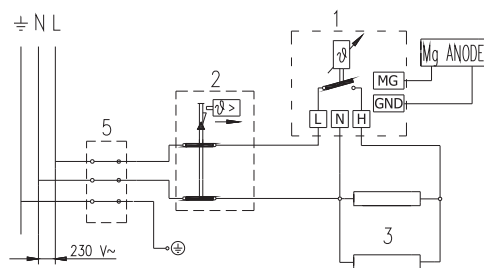
Електросхема
