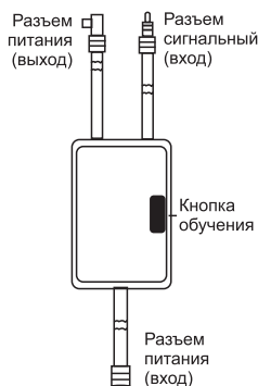
Внешний передатчик
