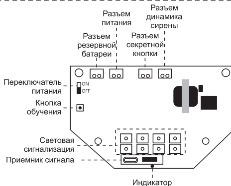
Плата сирены
