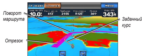
Следование маршруту на экране Mariner's Eye 3D
