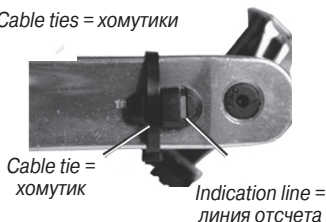
Рис.: Датчик GSC 10 на задней опоре цепи.
