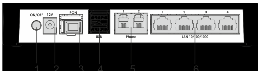
Рисунок 3 – Внешний вид задней панели NTP-RG-1402G-W rev.C
