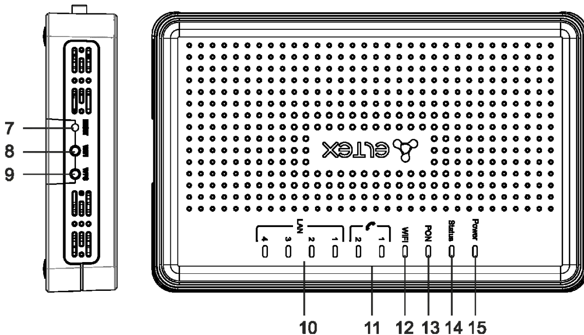
Рисунок 4 – Внешний верхней и боковой панели NTP-RG-1402G-W rev.C
