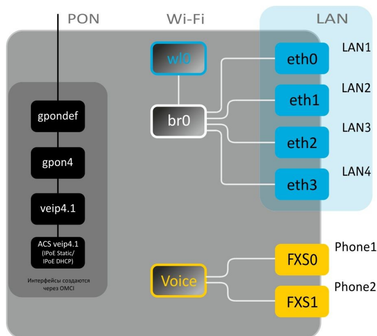
Рисунок 5 – Архитектура устройства с заводской конфигурацией
