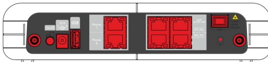
Рисунок 4 – Внешний вид задней панели NTE-RG-1402G-W rev.B
