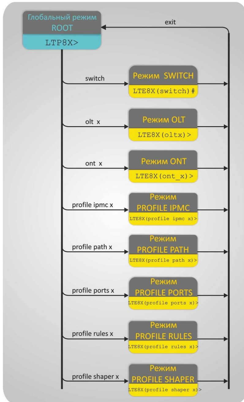
Рисунок 18 – Верхний уровень иерархии режимов команд
