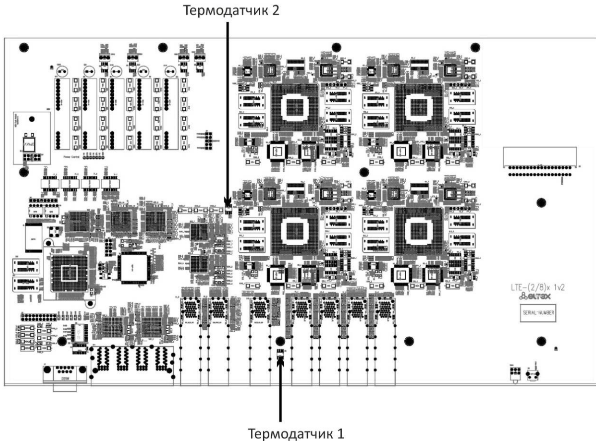
Рисунок 5 – Расположение термодатчиков
