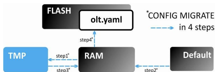
Рисунок 17 – порядок выполнения команды MIGRATE
