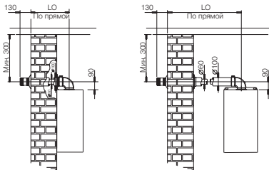
Горизонтальный коаксиальный дымоход
