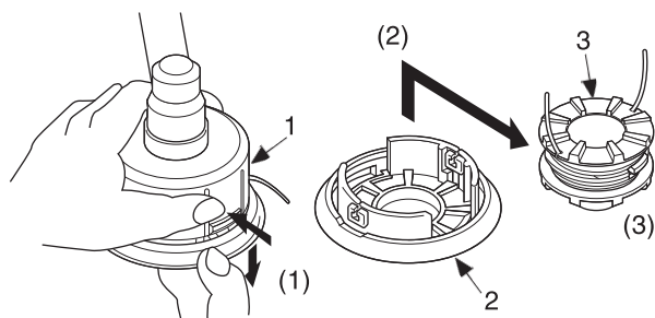
1. Корпус 2. Крышка
