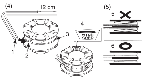
1. Изогнутая часть 2. Паз для нейлоновой лески 3. Промежуточный разделитель
