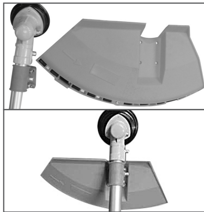
Рис. 2 Установка защитного кожуха
