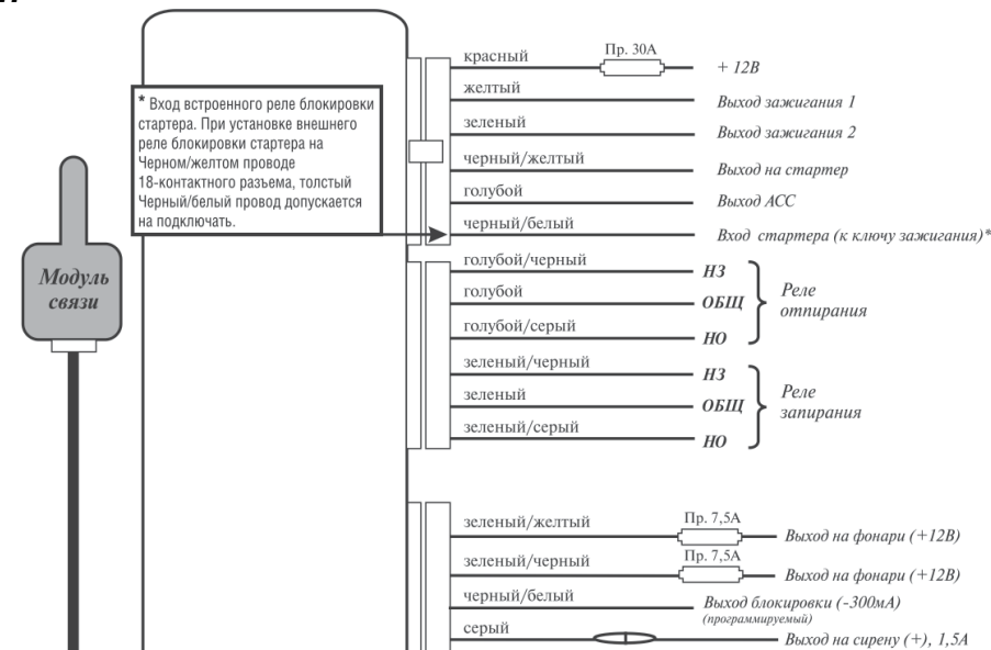
СХЕМА ПОДКЛЮЧЕНИЙ
