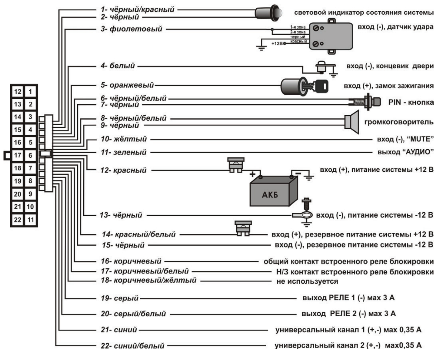
Схема подключения CARFON
