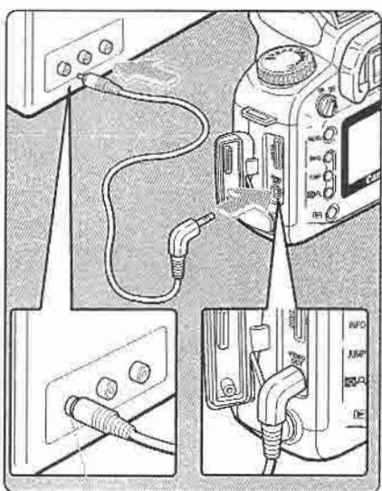
Разъем видеовхода
