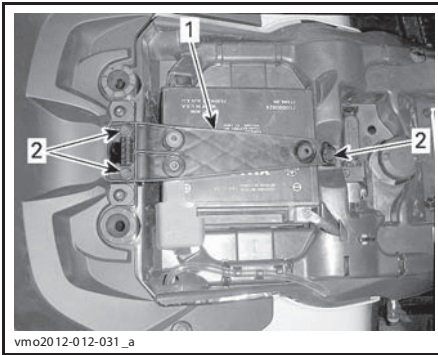
1. Ремень крепления аккумуляторной батареи 2. Винты крепления
