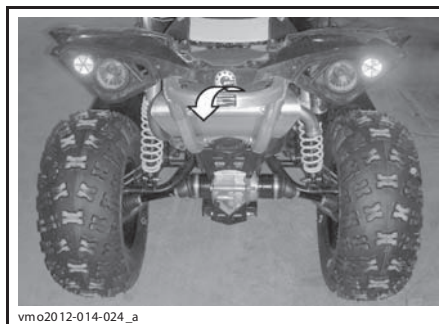
ТИПОВОЙ ВАРИАНТ — МЕСТО КРЕПЛЕНИЯ ЗАДНЕЙ ЧАСТИ МОТОВЕЗДЕХОДА
