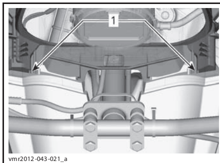
ДЛЯ НАГЛЯДНОСТИ НЕКОТОРЫЕ КОМПОНЕНТЫ СНЯТЫ
