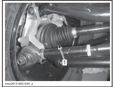
ЗАДНЯЯ ЧАСТЬ МОТОВЕЗДЕХОДА 1. Чехол наружного шарнира приводного вала
