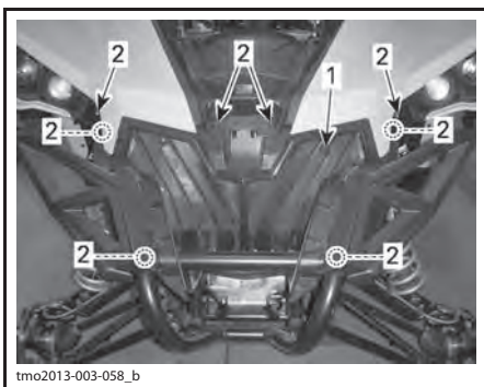
1. Пластмассовая крышка радиатора 2. Болты
