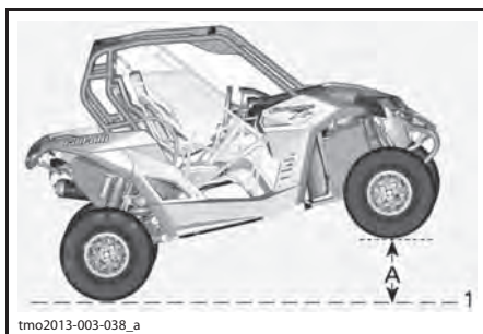
ПЕРЕДНЯЯ ЧАСТЬ МОТОВЕЗДЕХОДА ПОДНЯТА 1. Уровень опорной поверхности А. 65 см
