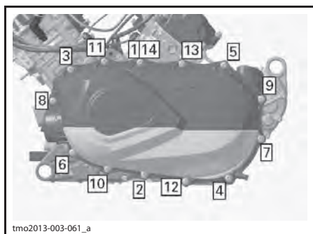
tmo2013-003-061_a ПОСЛЕДОВАТЕЛЬНОСТЬ ЗАТЯЖКИ ВИНТОВ КРЕПЛЕНИЯ КРЫШКИ ВАРИАТОРА
