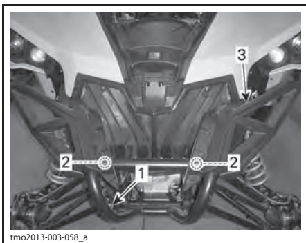
1. Нижний болт 2. Верхние болты 3. Бампер
