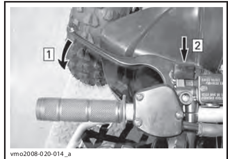
ЛЕВЫЙ РЫЧАГ ТОРМОЗА Шаг 1: Нажать и удерживать рычаг тормоза Шаг 2: Надавить на замок
