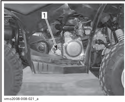
ТИПОВОЙ ВАРИАНТ — ПРАВАЯ СТОРОНА ДВИГАТЕЛЯ 1. Щуп
