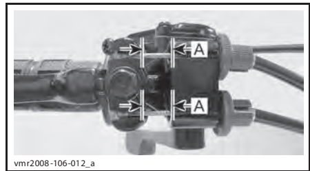
A. 10...12 мм
