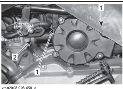
1. Снятие воздушного фильтра
