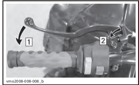
ТИПОВОЙ ВАРИАНТ — ЛЕВЫЙ РЫЧАГ ТОРМОЗА Шаг 1: Нажать и удерживать рычаг тормоза Шаг 2: Блокировочный рычажок
