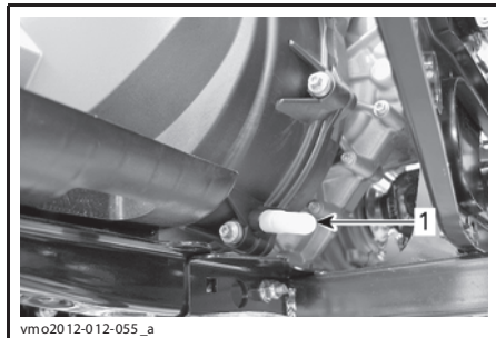
1. Дренаж вариатора
