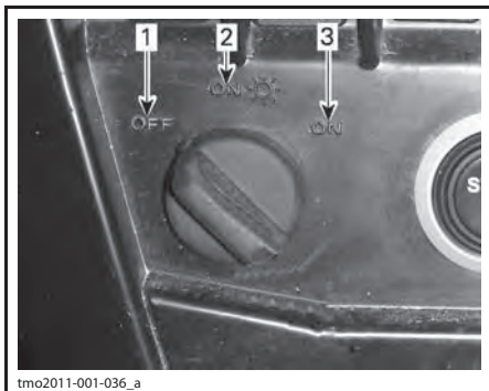
ПОЛОЖЕНИЕ ЗАМКА ЗАЖИГАНИЯ
