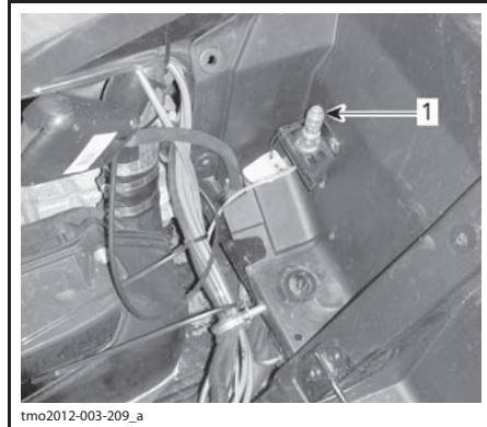
1. Штуцер компрессора
