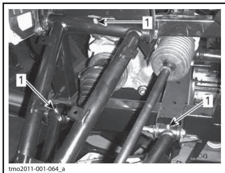
ПЕРЕДНЯЯ ПОДВЕСКА — ТИПОВОЙ ВАРИАНТ 1. Пресс-масленки
