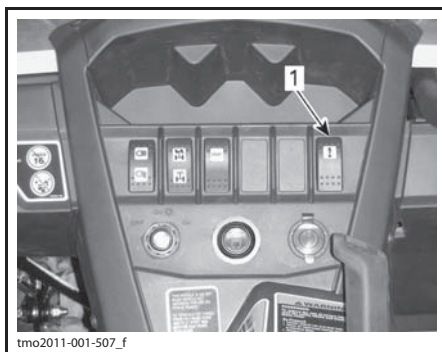
1. Переключатель лебёдки
