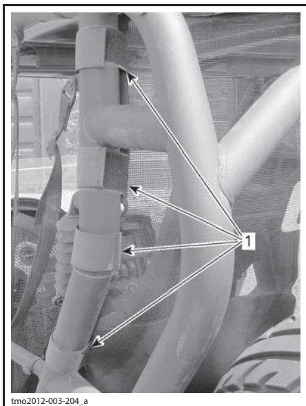
ТИПОВОЙ ВАРИАНТ — ЛЕВАЯ СТОРОНА 1. Стропы
