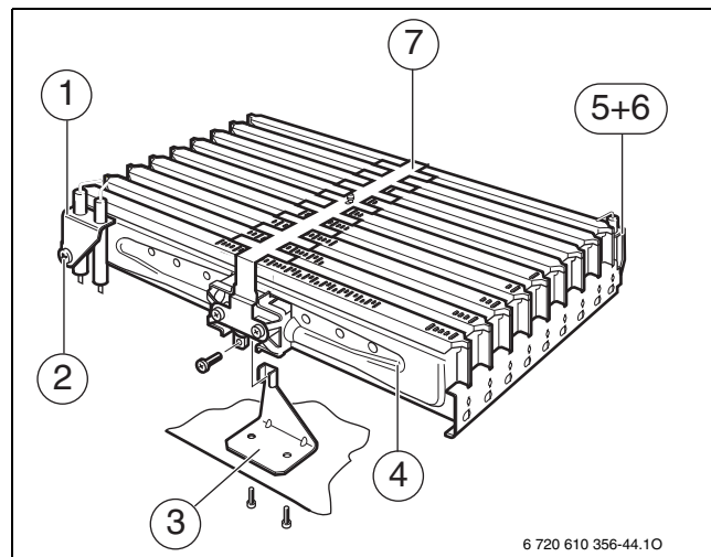
Рис 75 Узел горелки
