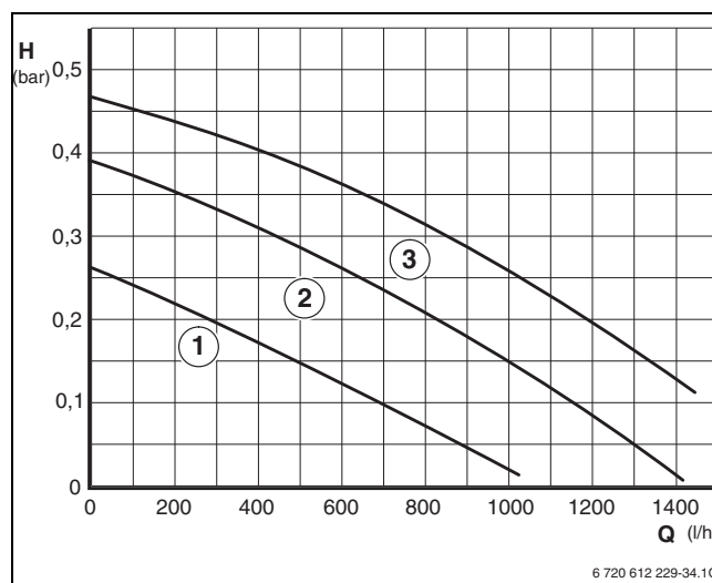
Рис 25 Характеристики насоса
