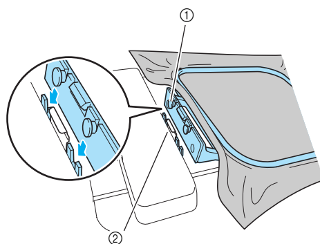
① Направляющие язычки пялец
