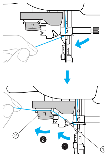
① Выемка нитенаправителя
