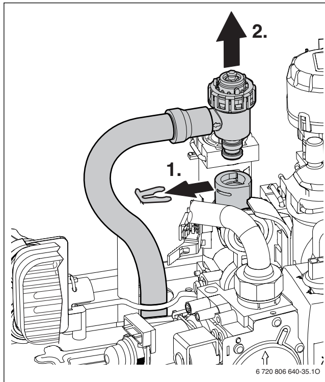
Рис. 36 Демонтаж предохранительного клапана (отопительного контура)
