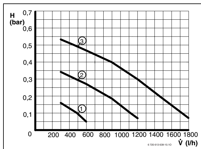
Рис 29 Характеристики насоса
