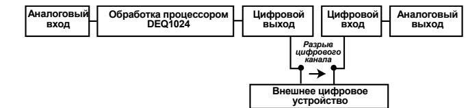
Рисунок 2.6: Прохождение сигнала в режиме POST EQ
