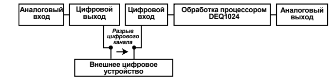
Рисунок 2.5: Прохождение сигнала в режиме PRE EQ
