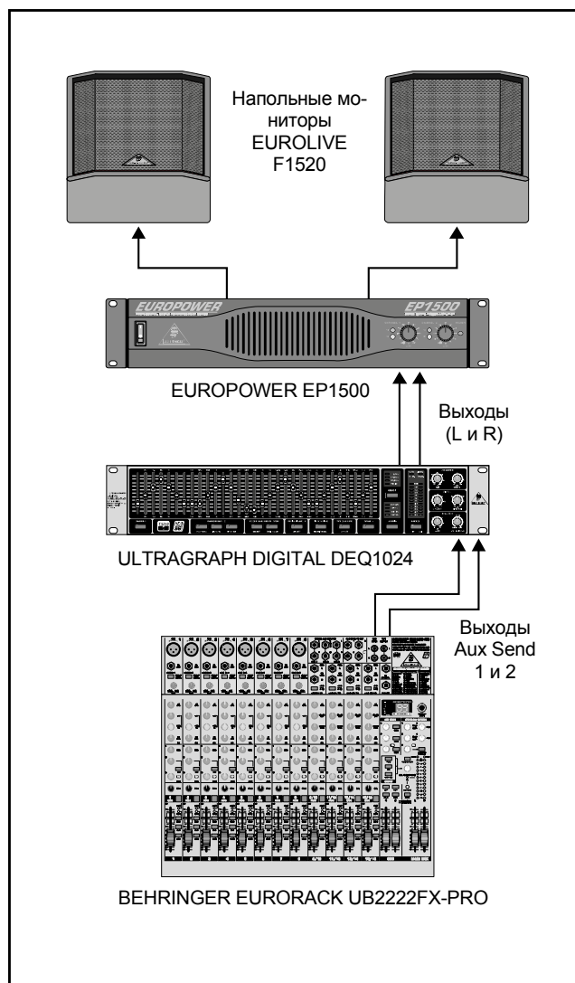
Рисунок 3.2: Применение процессора ULTRAGRAPH DIGITAL DEQ1024 в системе мониторов
