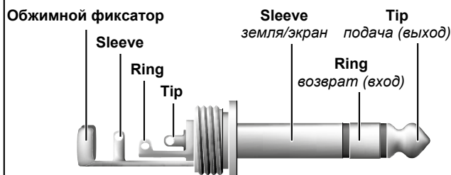
Рисунок 4.4: Штекер разъема TRS ¼ дюйма для применения в цепи разрыва канала при подаче/возврате сигнала с внешнего устройства
