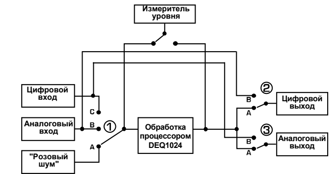
Рисунок 2.4: Соединения входного/выходного сигнала в зависимости от режима работы процессора DEQ1024
