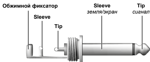
Рисунок 4.2: Штекер разъема TS ¼ дюйма
