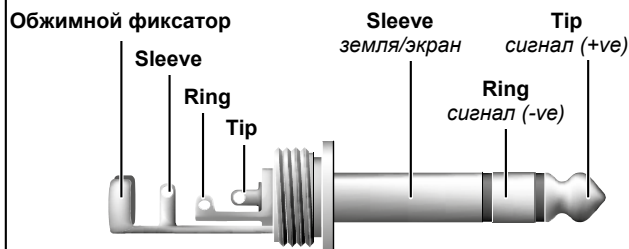
Рисунок 4.3: Штекер разъема TRS ¼ дюйма
