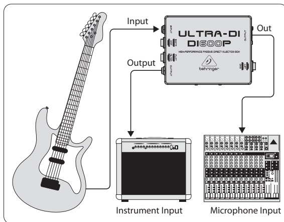
Fig. 2: Гитара → DI-бкс → гитарный усилитель/микшерный пульт
