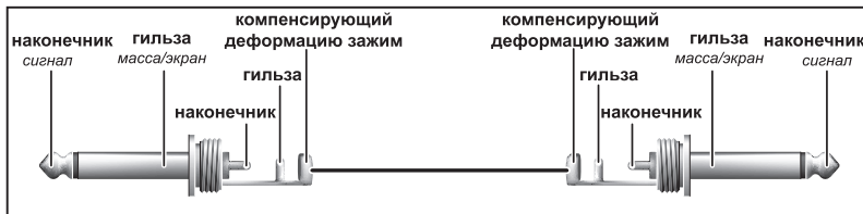
Рис. 5.1: Разводка инструментального кабеля
