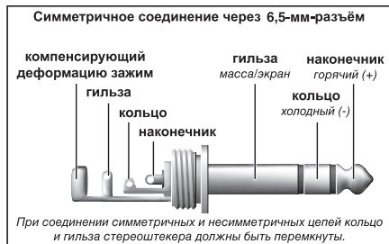
Рисунок 5.2: 6,3-мм-стереоштекер
