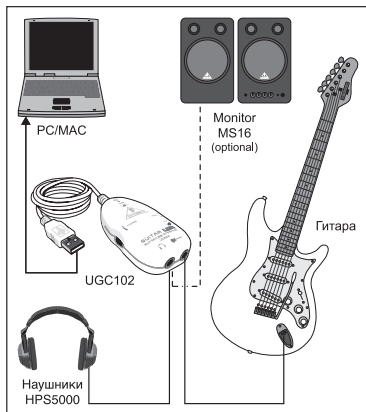
Рис. 4.1: Подключение UCG102
