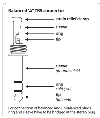
Рис. 4.2: 6,3 мм-стереоштекер
