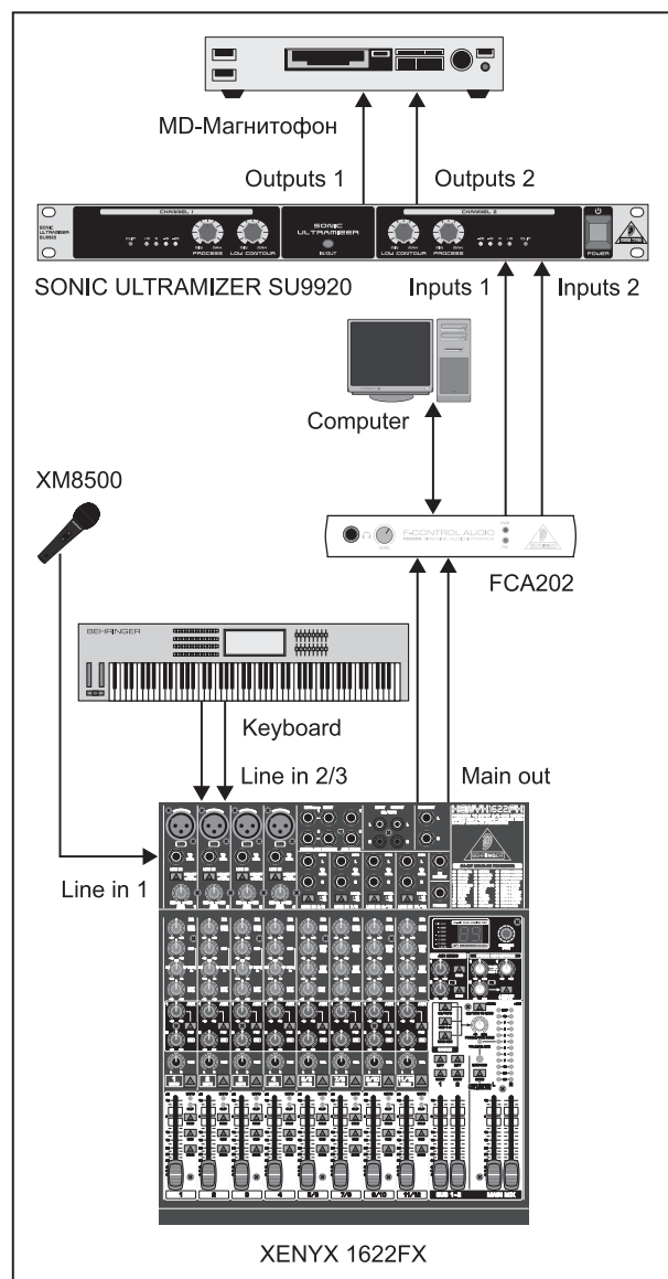
Рис. 3.2: Работа с SU9920 в студии
