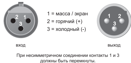
Рис. 4.3: Симметричный XLR-штекер
