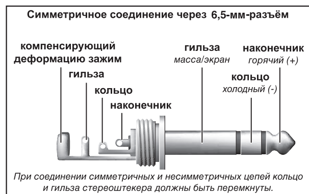
Рис. 4.2: Симметричный кабель со стереоштекерами.
