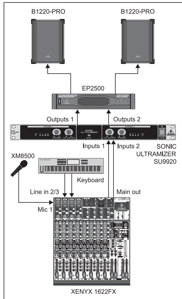
Рис. 3.1: Работа SU9920 с системами озвучения
