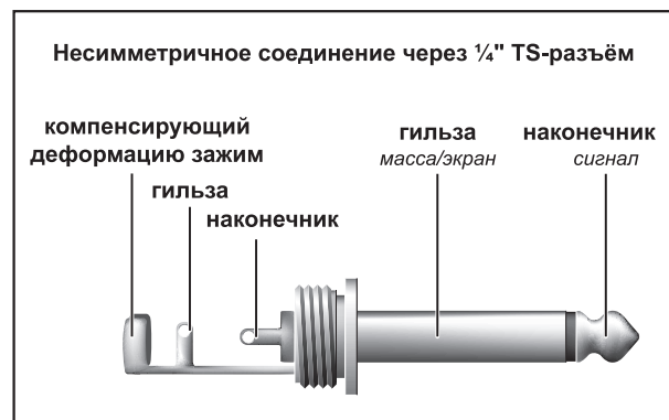
Рис. 4.1: Асимметричный кабель с моноштекерами
