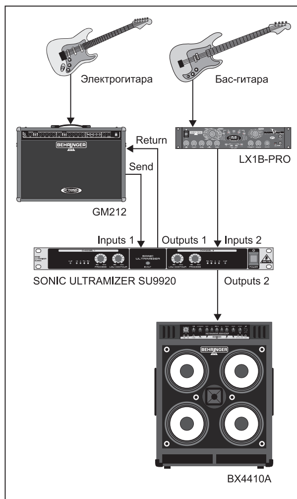
Рис. 3.3: Работа SU9920 с гитарными усилителями
