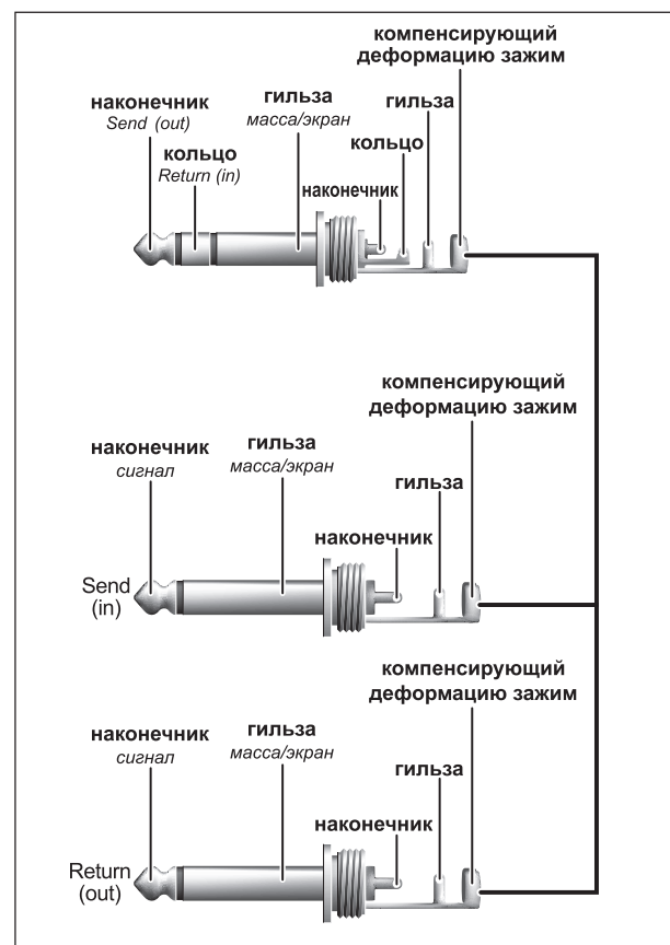
Рис. 4.4: Insert-кабель с одним стерео- и двумя моноштекерами
