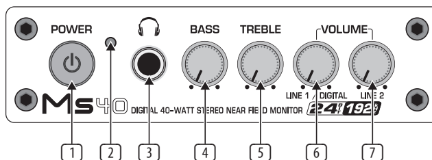
Рис. 2.1: Передняя панель, элементы управления (правая колонка)
