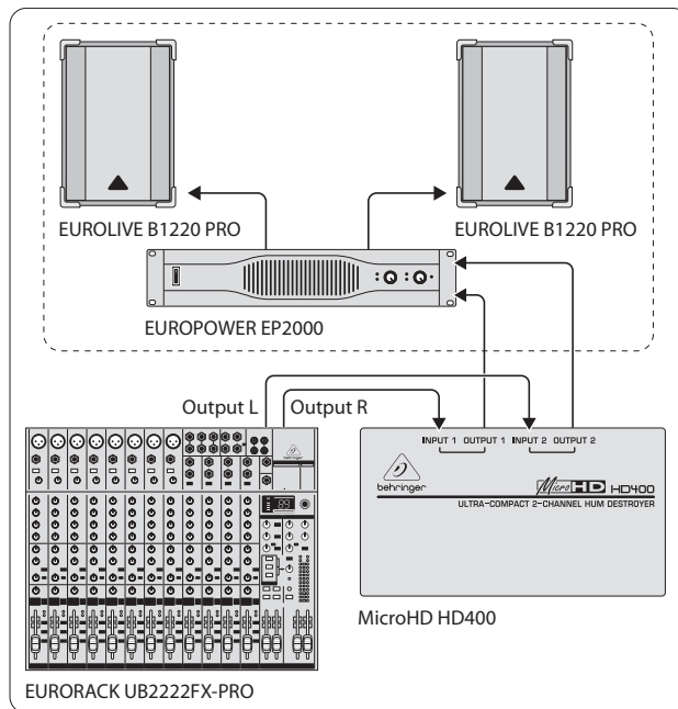
Каблирование HD400
