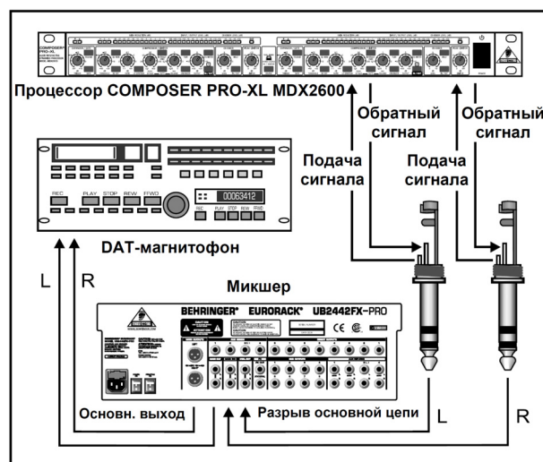
Рисунок 4.2: Компрессия основного смешанного сигнала с помощью процессора MDX2600
