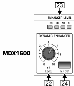
Рисунок 2.4: Элементы управления секции динамического энхансера
