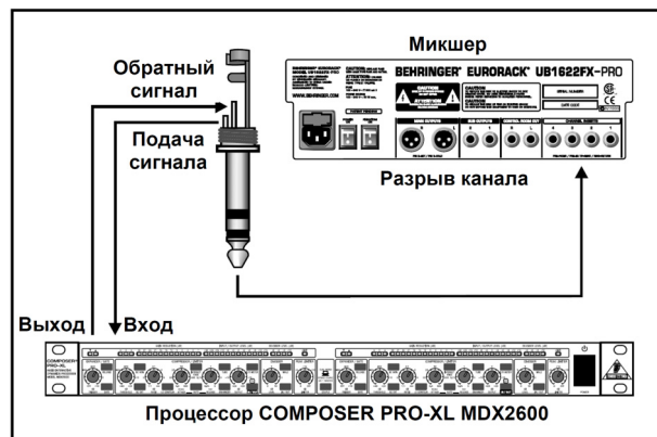
Рисунок 4.1: Подключение динамического процессора в разрыв цепи канала
