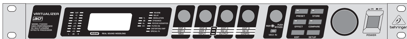
Рис. 1.1: Передняя панель VIRTUALIZER 3D
