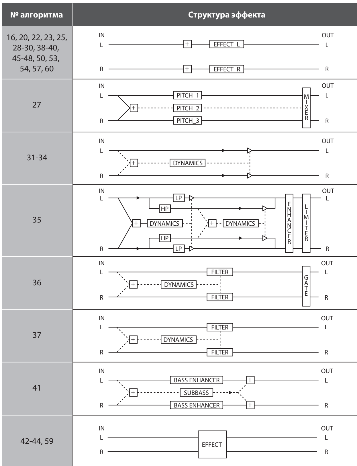
Рис.3.2: Структура эффектов, часть 2
