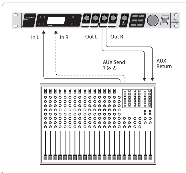
Рис. 4.1: Соединение аух-шин
