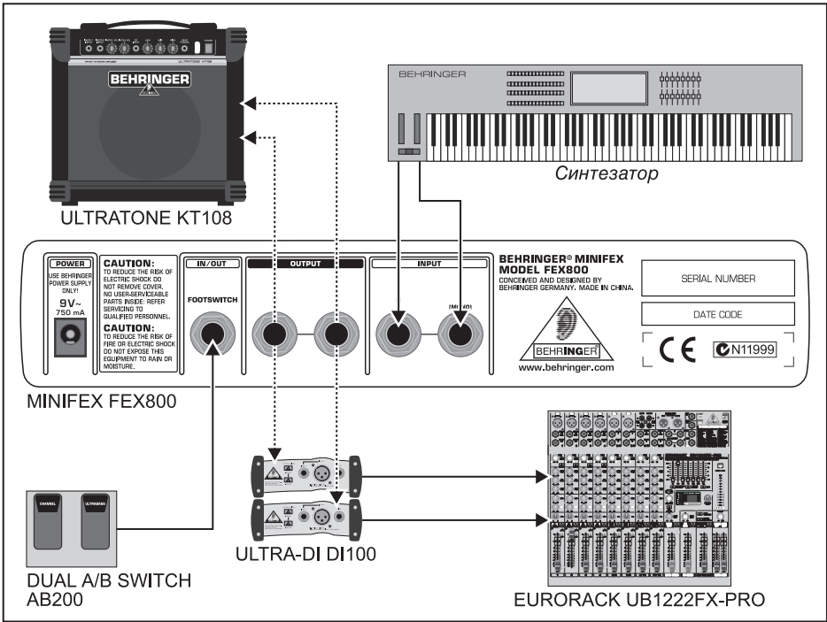
Рис. 4.3: Пример подключения MINIFEX к усилителю или к DI-боксу
