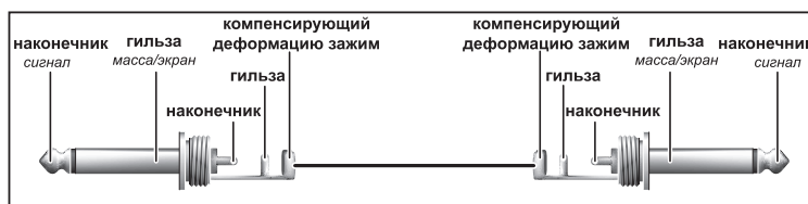
Рис. 5.2: Несимметричный кабель с 6,3 мм-моноштекерами
