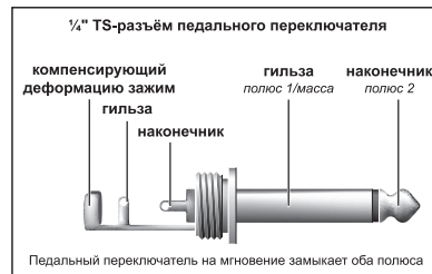
Рис. 5.3: 6,3 мм-моноштекер для подключения педали
