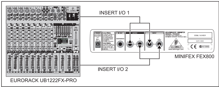
Рис. 4.2: Подключение MINIFEX к каналным разрывам
