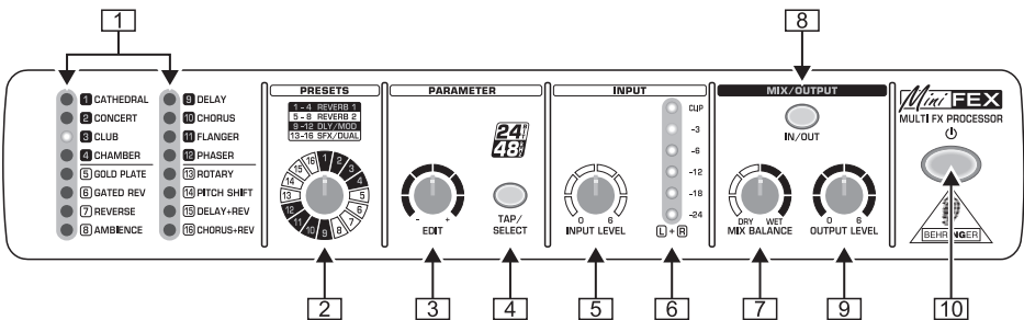
Рис. 2.1: Передняя панель FEX800, элементы управления
