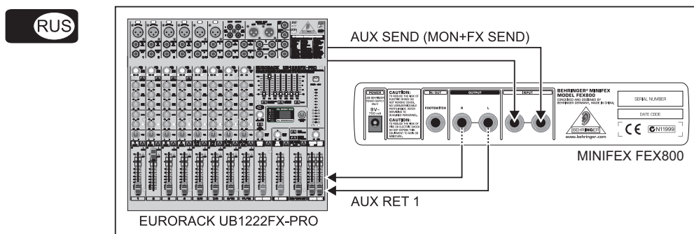
Рис. 4.1: Подключение MINIFEX к Aux-тракту
