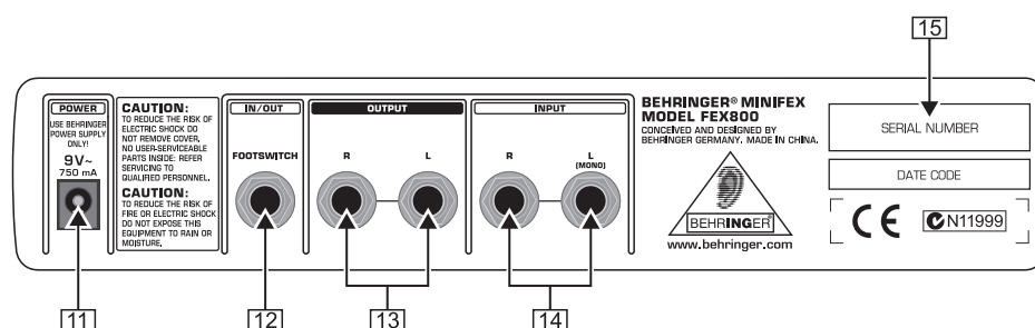
Рис. 2.2: Задняя панель FEX800
