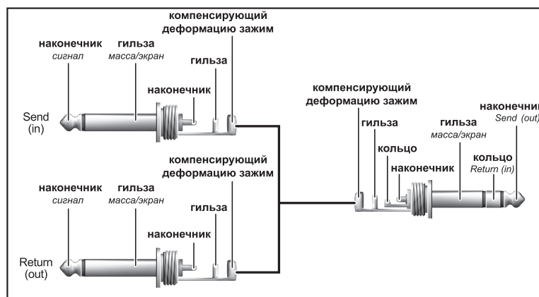
Рис. 5.1: Insert-кабель с одним стерео- и двумя моноштекерами
