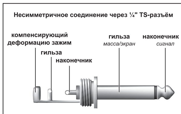
Рисунок 4.1: 6,3-мм-моноштекер
