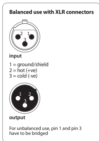
Рис. 4.3: XLR-соединения
