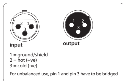
Рисунок. 4.3: XLR-соединения
