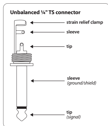
Рисунок 4.1: 6,3-мм-моноштекер
