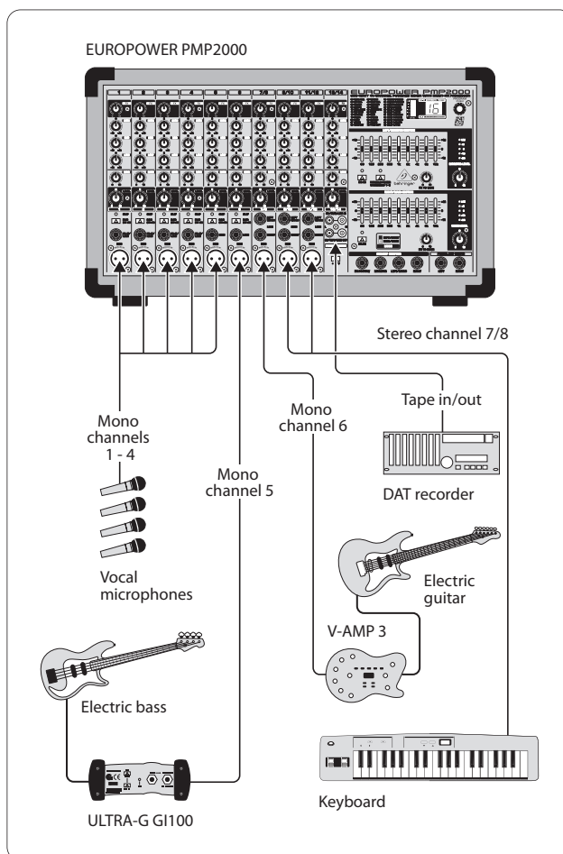
Рисунок 5.3: Стандартное исполнение (пример)
