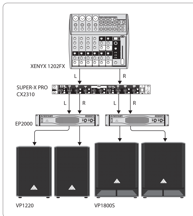
Фиг. 5.3: Двухканальный стерефонический режим с субвуферами
