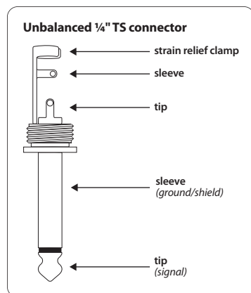
Фиг. 2.3: Разъем TS громкоговорителя размером ¼ дюйма.
