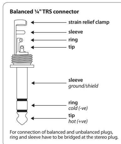
Рис. 4.1: 6,3-мм TRS-штекер
