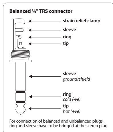
Рис. 4.1: 6,3-мм TRS-штекер
