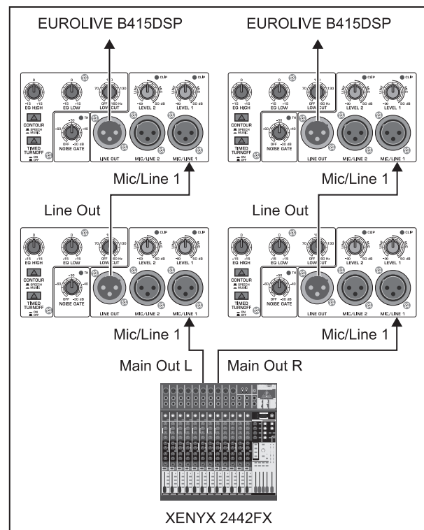
Рис. 3.3: Соединение нескольких B415DSP
