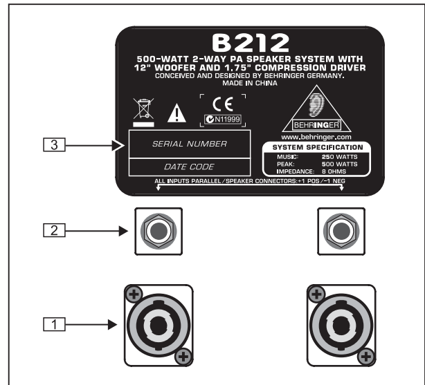
Рис. 2.1. Разъемы (B212 и B215)
