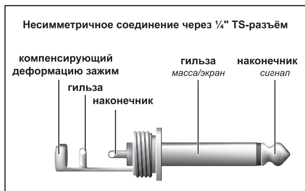
Рис. 6.2: 6,3-мм моноштекер
