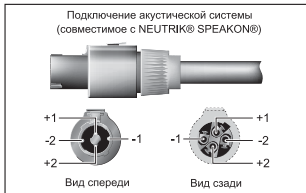
Рис. 6.1: Штекер Speakon®
