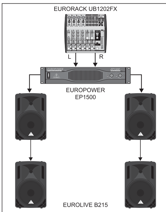
Рис. 5.2. Коммутация нескольких B212/B215
