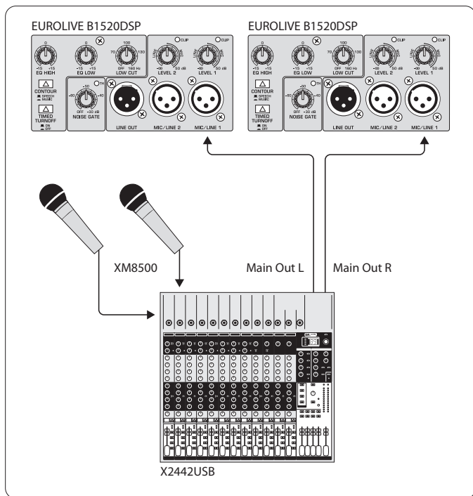
Рис. 3.2: Подключение микшерного пульта
