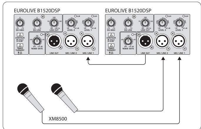
Рис. 3.1: Подключение микрофонов
