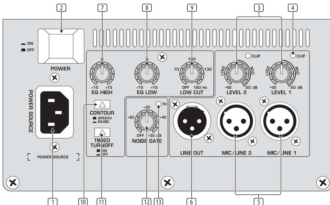
Рис. 2.1: Обратная сторона, элементы управления и разъемы
