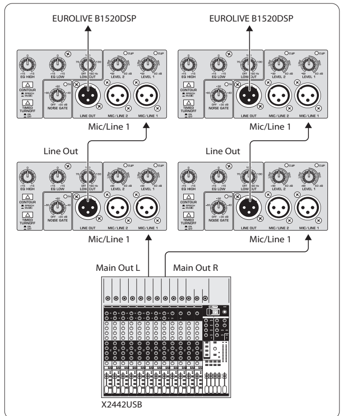
Рис. 3.3: Соединение нескольких B1520DSP
