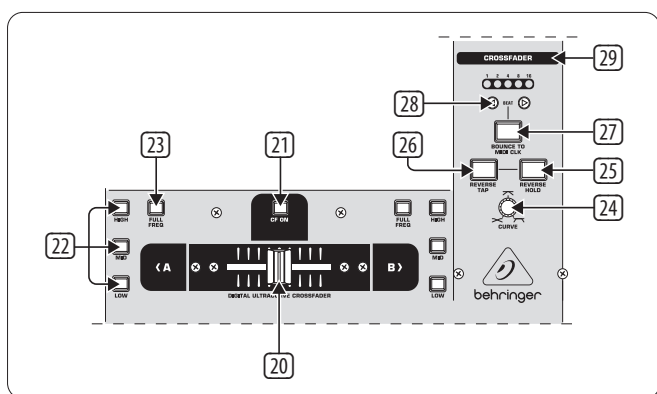
Рис. 2.3: Секция кроссфейдера
