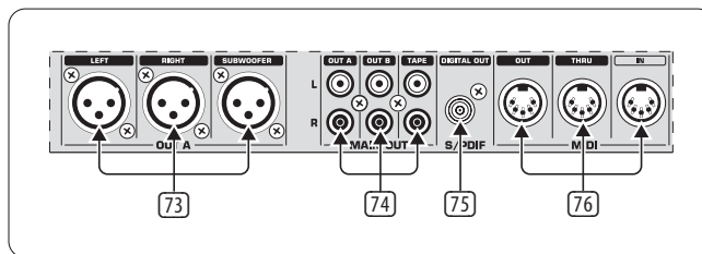
Рис. 2.8: Выходы DDM4000
