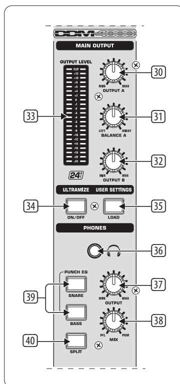
Рис. 2.4: Секция Main / Phones
