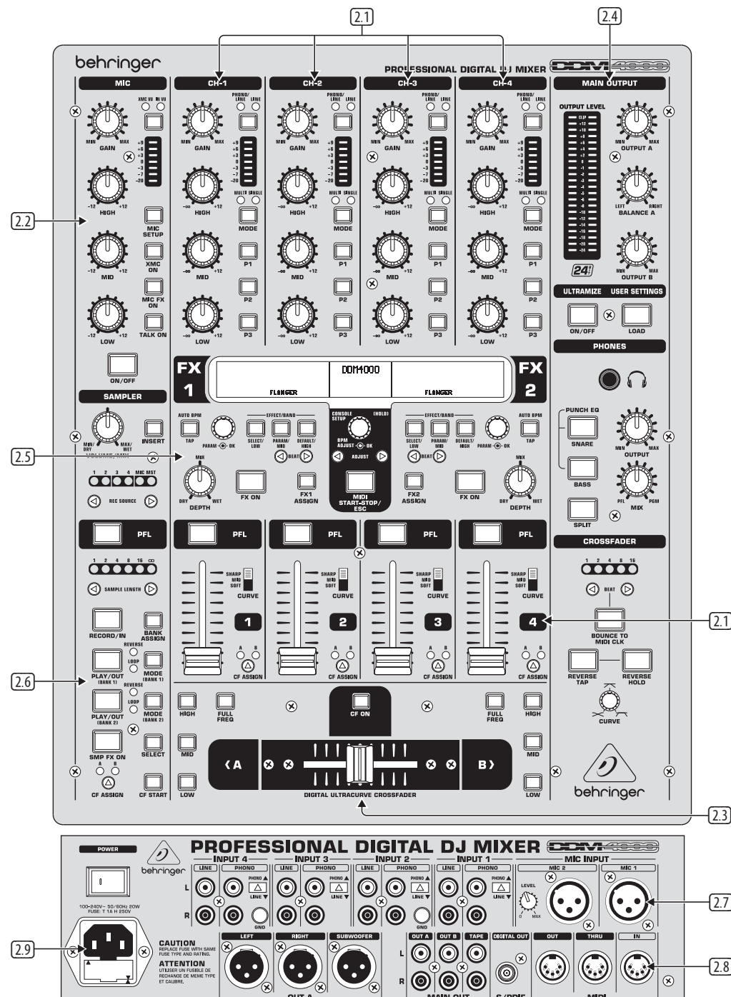
Рис. 2.0: общий вид DDM4000
