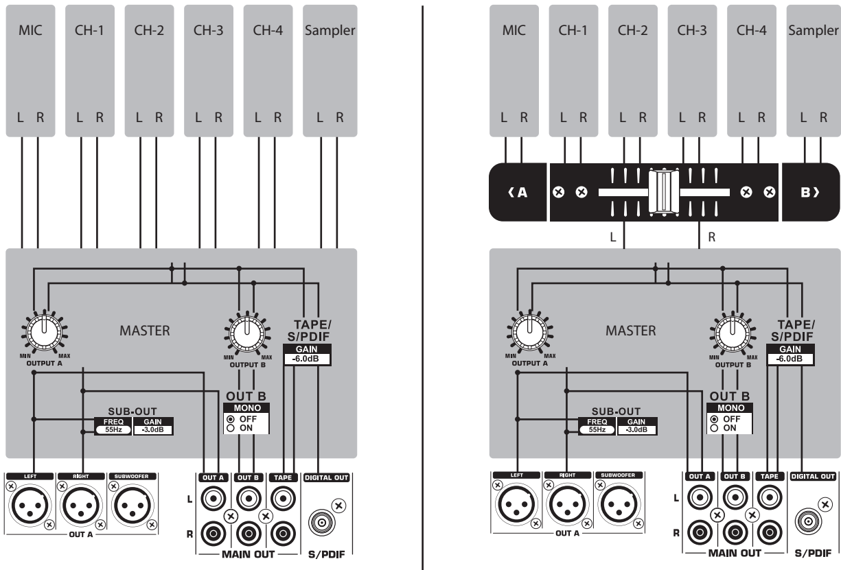
Fig. 10.2: Примеры маршрутизации микшера
