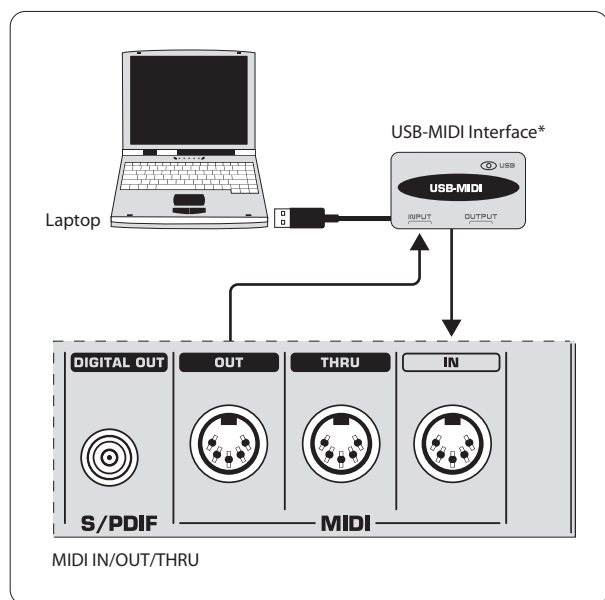
Рис. 7.1: Подключение DDM4000 к компьютеру
