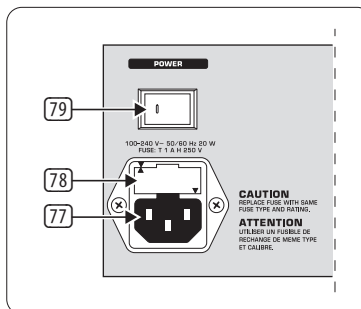
рис. 2.9: Секция POWER
