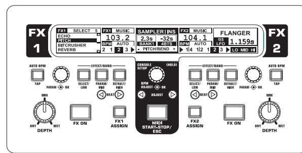
Рис. 4.1: Секция BPM и эффектов
