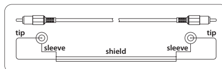
Рис. 8.3: RCA-кабель
