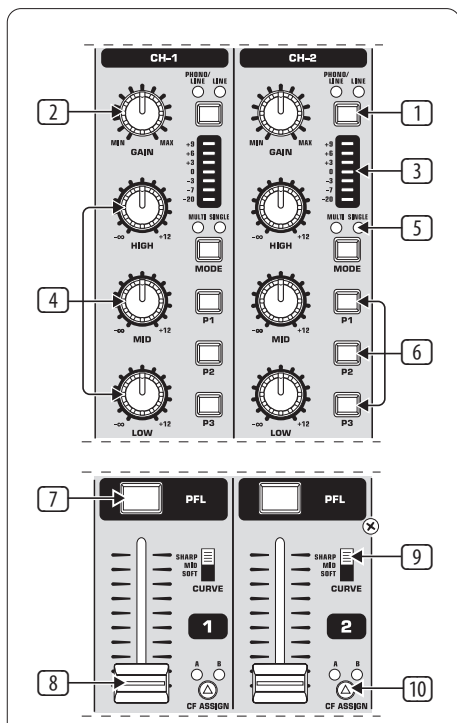
Рис. 2.1: Стереоканалы
