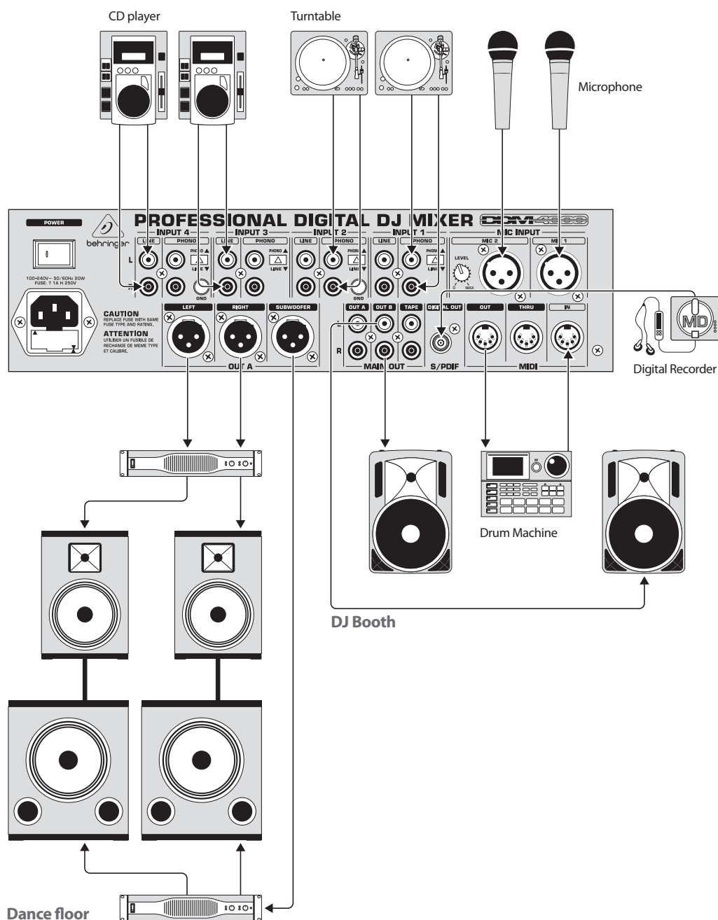
Рис. 2.10: Пример подключения DDM4000
