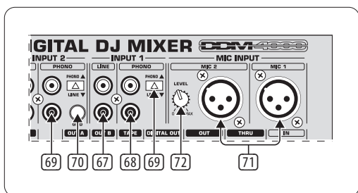
Рис. 2.7: Входы DDM4000
