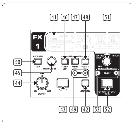
Рис. 4.2: Секция эффектов (здесь: FX 1)
