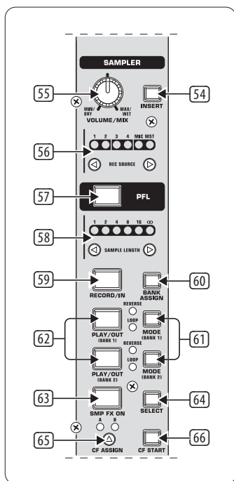
Рис. 5.1: Секция сэмплера
