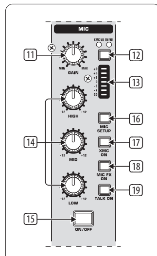
Рис. 2.2: Микрофонный канал
