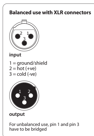
Рис. 8.1: XLR-соединения
