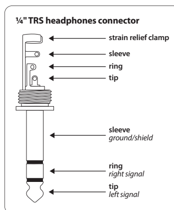
Рис. 8.2: Разъем наушников
