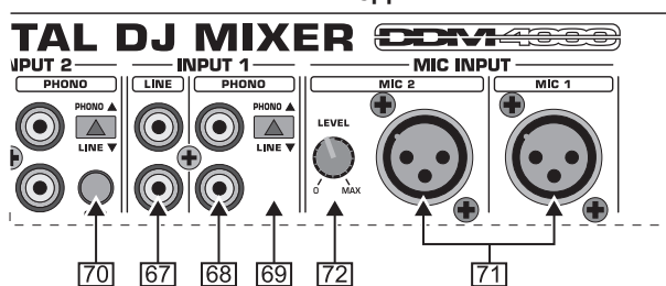
Рис. 2.7: Входы DDM4000
