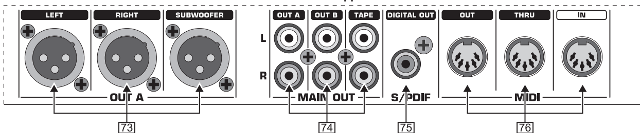
Рис. 2.8: Выходы DDM4000
