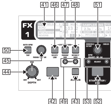
Рис. 4.2: Секция эффектов (здесь: FX 1)
