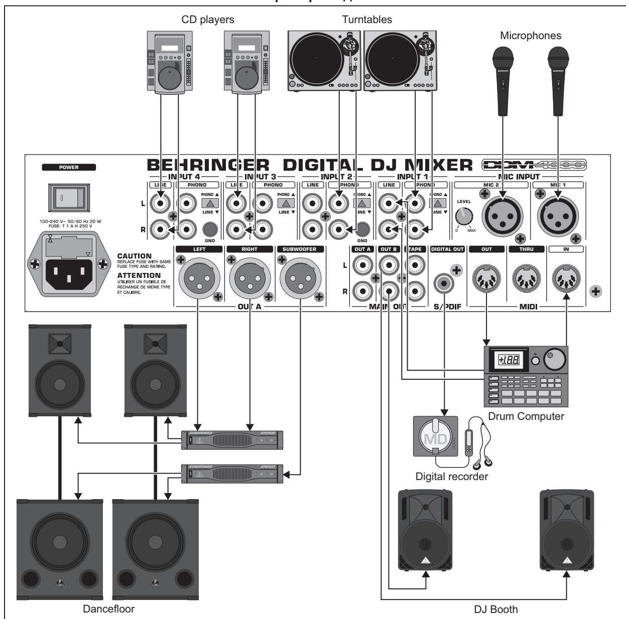
Рис. 2.10: Пример подключения DDM4000
