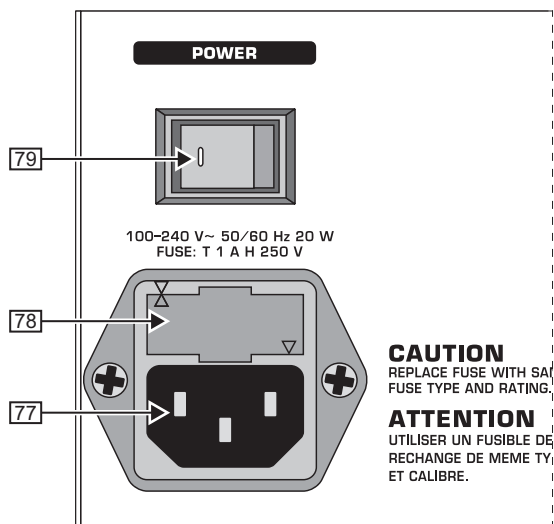
Рис. 2.9: Секция POWER
