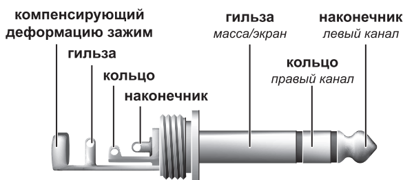
Рис. 8.2: Разъём наушников
