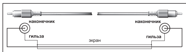
Рис. 8.3: RCA-кабель
