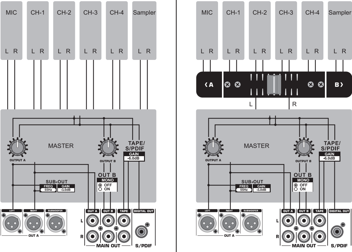
Рис. 10.2: Примеры маршрутизации микшера
