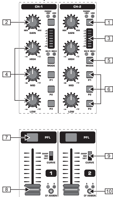
Рис. 2.1: Стереоканалы
