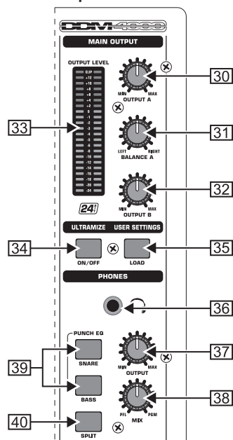
Рис. 2.4: Секция Main / Phones
