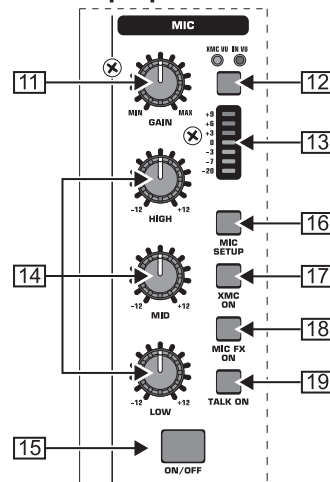
Рис. 2.2: Микрофонный канал
