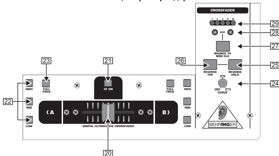
Рис. 2.3: Секция кроссфейдера
