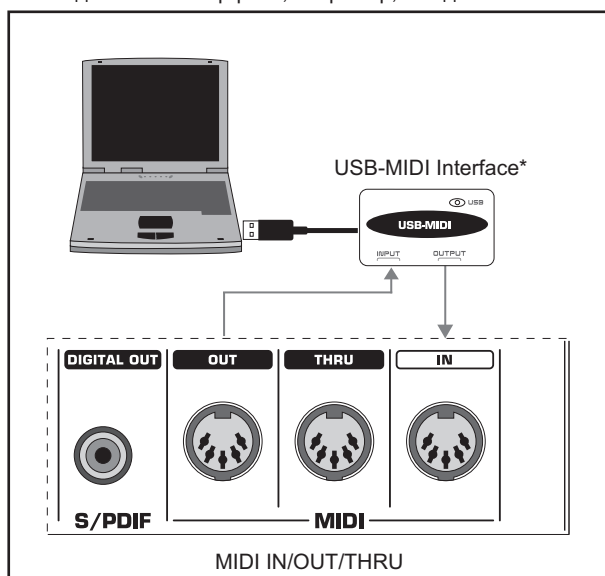
Рис. 7.1: Подключение DDM4000 к компьютеру
