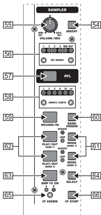
Рис. 5.1: Секция сэмплера
