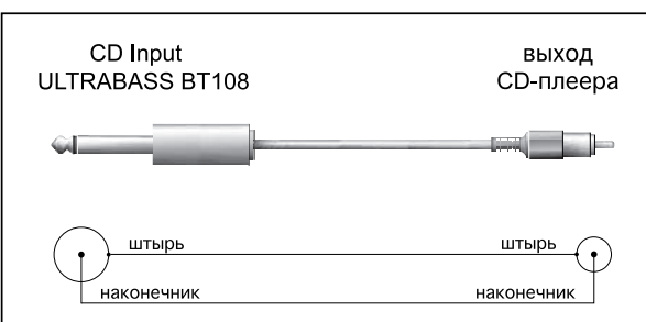
Рис. 4.4: Адаптерный монокабель
