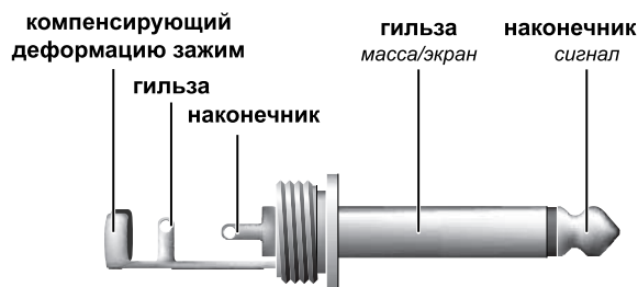
Рис. 4.1: Монофонический штепсель для гнезда INSTRUMENT INPUT
