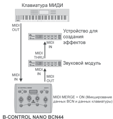
Рис. 3.2: Контроллер аппаратных средств
