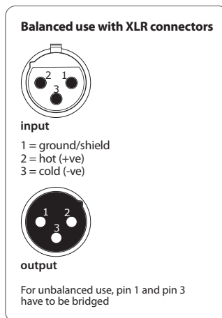
Рис. 6.1: Соединения XLR
